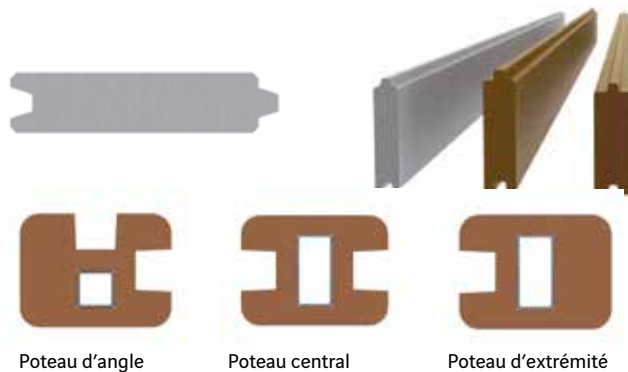
Poteau d'angle
